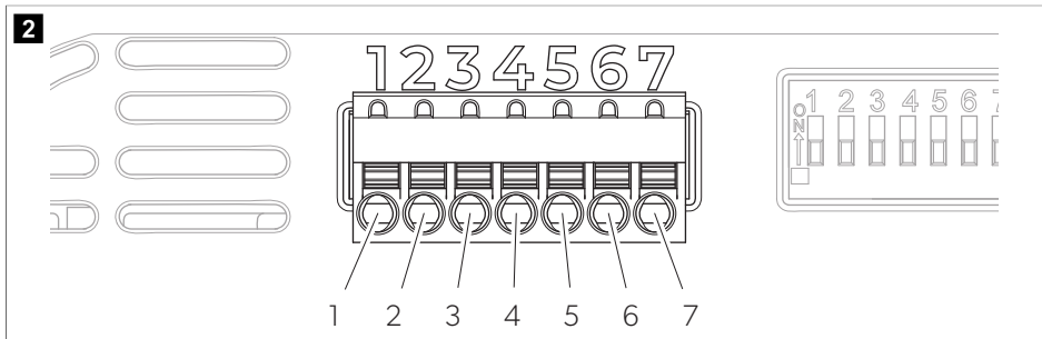
Taulu 133. Riviliitin
