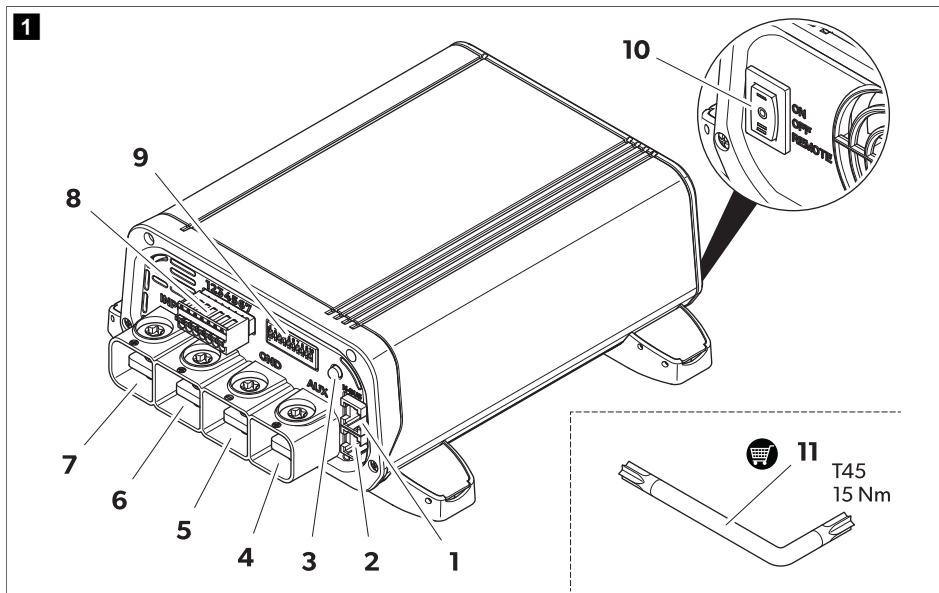
Taulu 131. Liitännät ja käyttölaitteet
