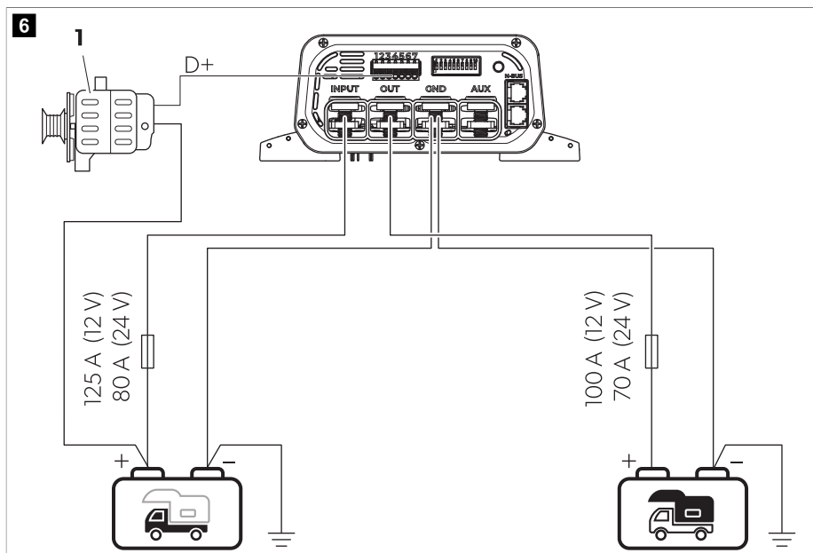
Tabulka 175: Diagram připojení, varianta A
