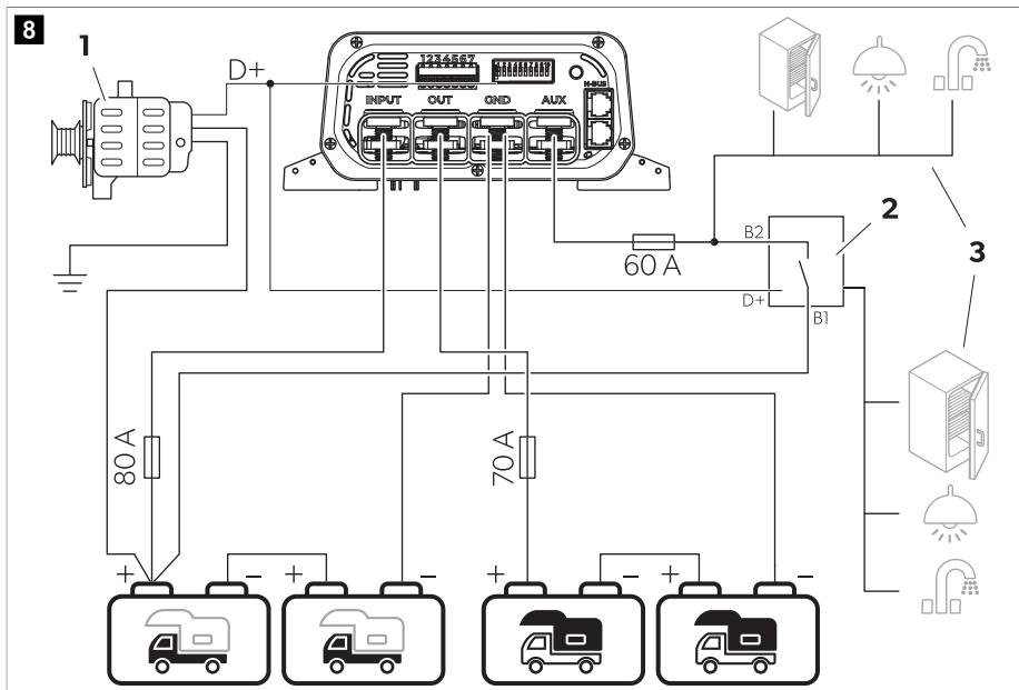
Taulu 138. Liitäntäkaaviomalli C
