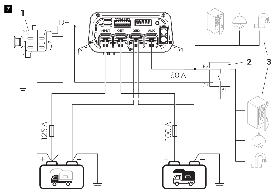
Πίνακας 280: Διάγραμμα συνδέσεων, παραλλαγή Β
