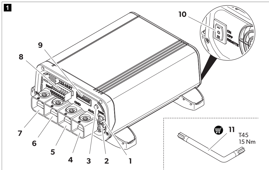
Tabula 300: Savienojumi un vadības opcijas
