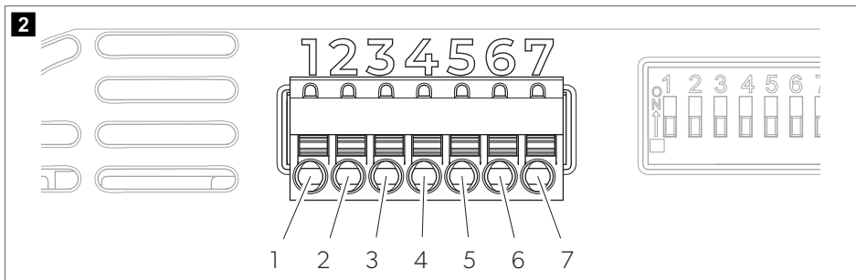
Tablica 198: Priključnica
