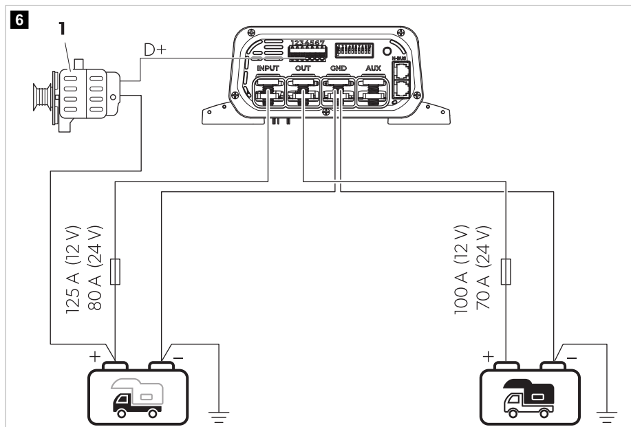
táblázat 188: 'A' csatlakoztatásirajz-változat
