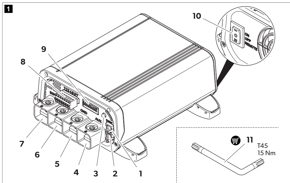
táblázat 183: Csatlakozók és kezelőelemek
