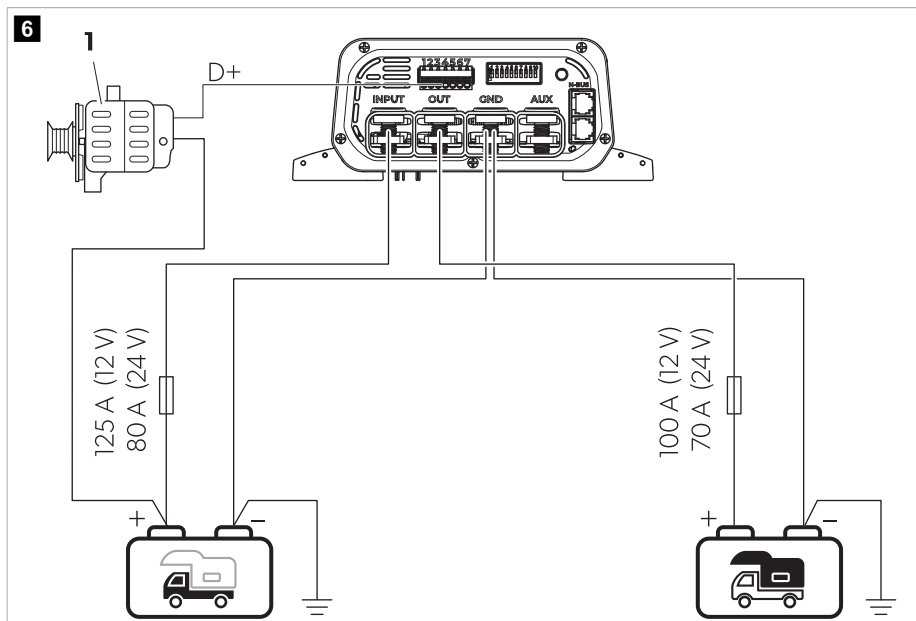
Tabula 305: Savienojuma shēmas variants A
