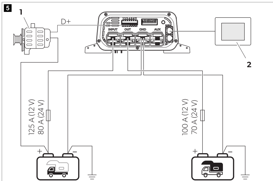
Tablica 200: Opća priključna shema
