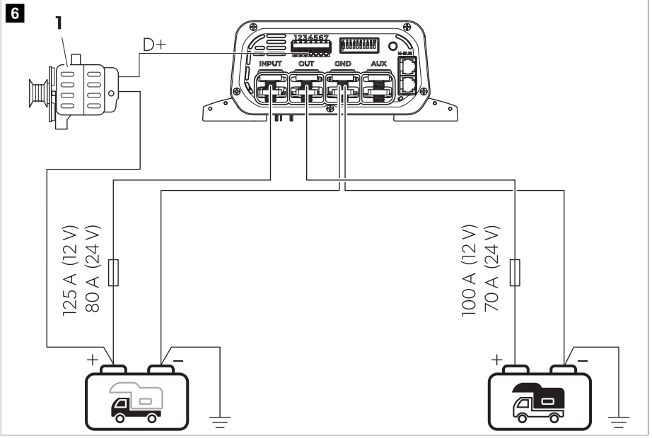
Çizelge 214: Bağlantı şeması tip A
