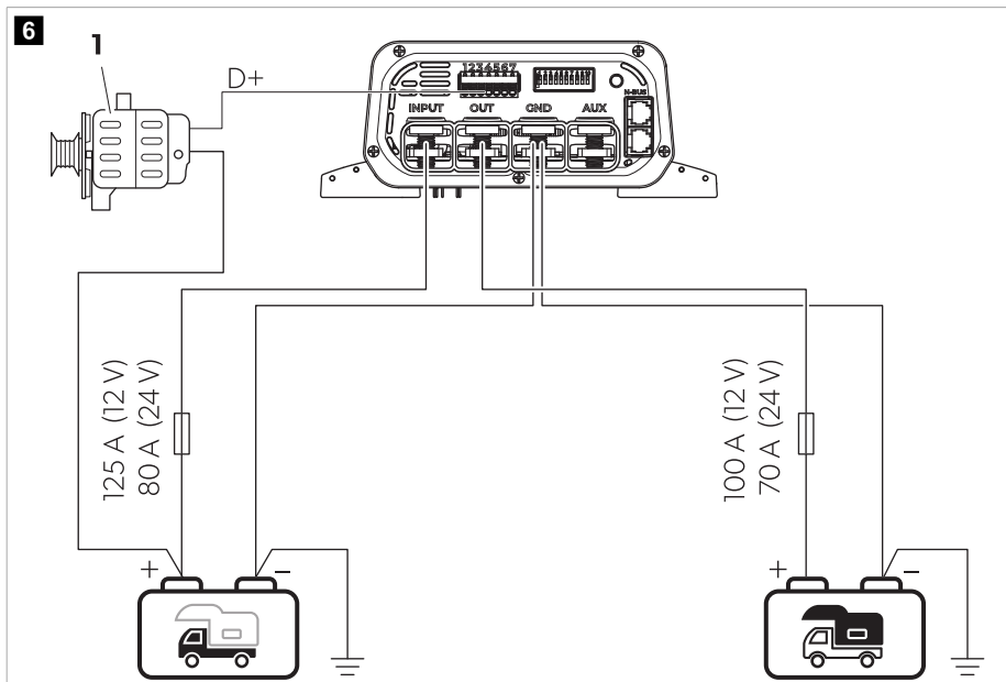
Taulu 136. Liitäntäkaaviomalli A
